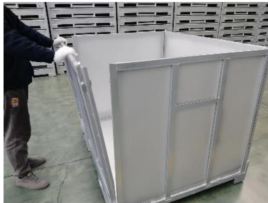
第二步： 把大门拉向自己
